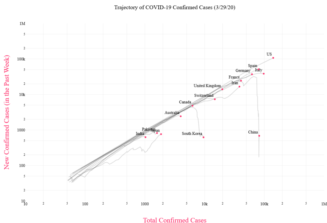
Figura 4. Representación de la trayectoria de la infección por SARS-CoV-2 en diversos países del mundo 8 .
