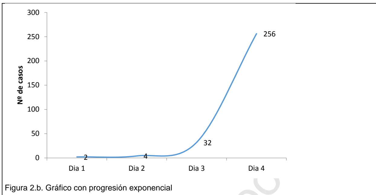
Figura 2. Gráficos simulados que representan un crecimiento lineal y un crecimiento exponencial.
